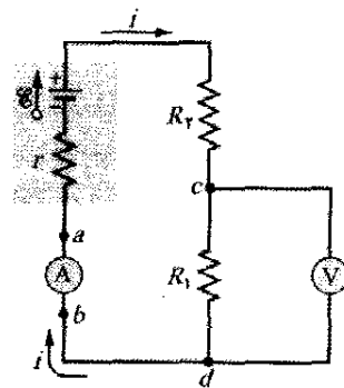
شکل ۲۳-۱۴ یک مدار تک حلقه‌ای که نشان می‌دهد آمپرسنج (A) و ولت‌سنج (V) چگونه در مدار قرار می‌گیرند.
